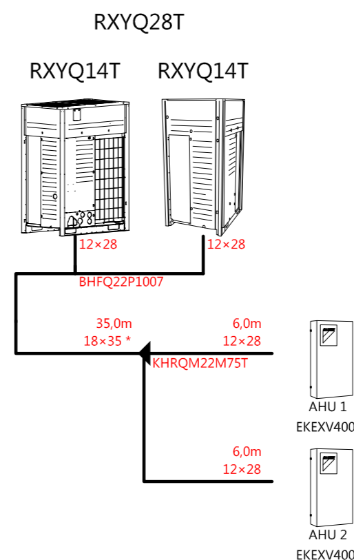
2 csöves VRV rendszer (2 körös DX utóhűtő/utófűtő)
